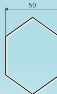
素線 線径3.0 mm
